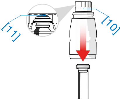
Inserimento dell'unità cuscinetto
