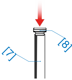
Unità cuscinetto sull'ausilio per il montaggio
