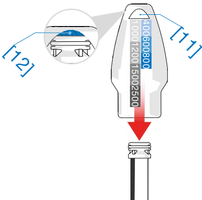
Insert rotor
